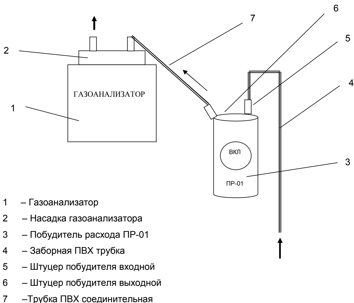
Рисунок 3.1 Схема забора и подачи пробы
